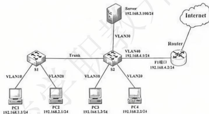
图 2 网络结构图
